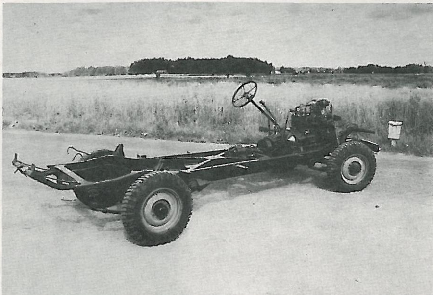
Terrängbilschassi.
